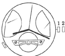
TY2505 (2505) 38 Jewels
